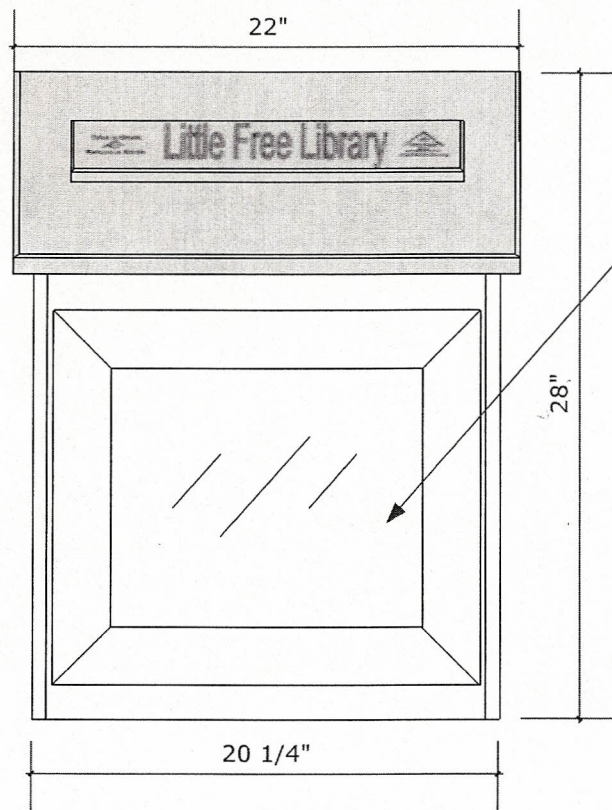
Front scale: 1 1/2"=1' A 03
