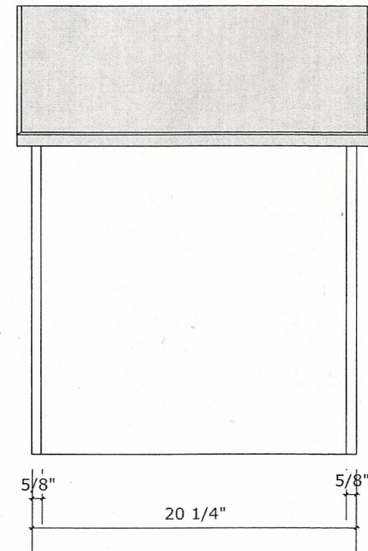
Back scale: 1 1/2"=1' C 03
